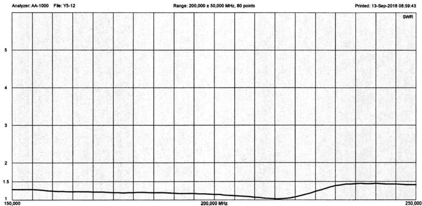
Współczynnik fali stojącej (VSWR) dla anteny Yagi 5-12 / 4-elementowej
